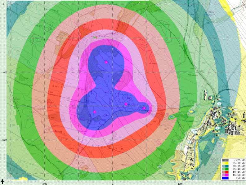
Příloha č. 7. STAV 2, výška pásem izofon 3 m n.t.
